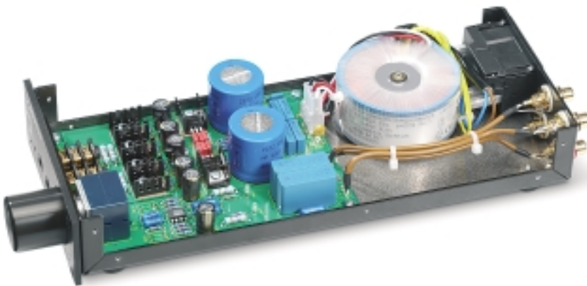
Die Dip-Schalter für die Wahl der Verstärkung befinden sich frei zugänglich an der Geräteunterseite. Der 30-Watt-Transformator ist magnetisch geschirmt
